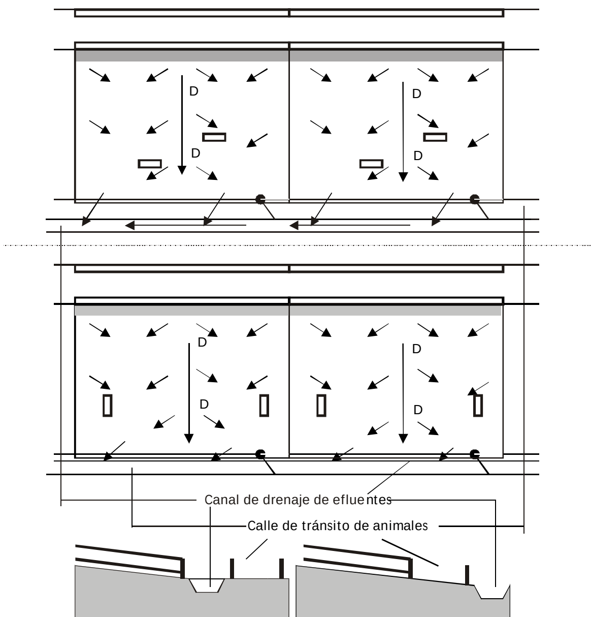
Diagrama del diseño del flujo de efluentes en escurrimiento superficial (NSW Agriculture, 1998).
