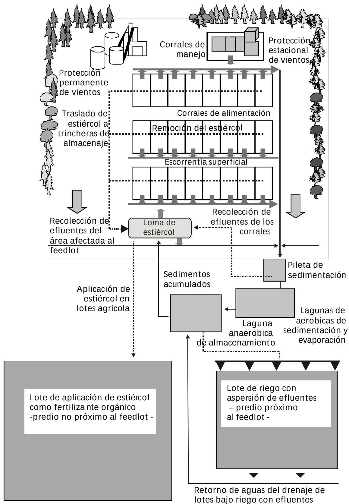
Figura 3.1. Esquema de una estructura de manejo de efluentes líquidos (circuito azul) y de estiércol (circuito marrón) en el diseño de un feedlot
