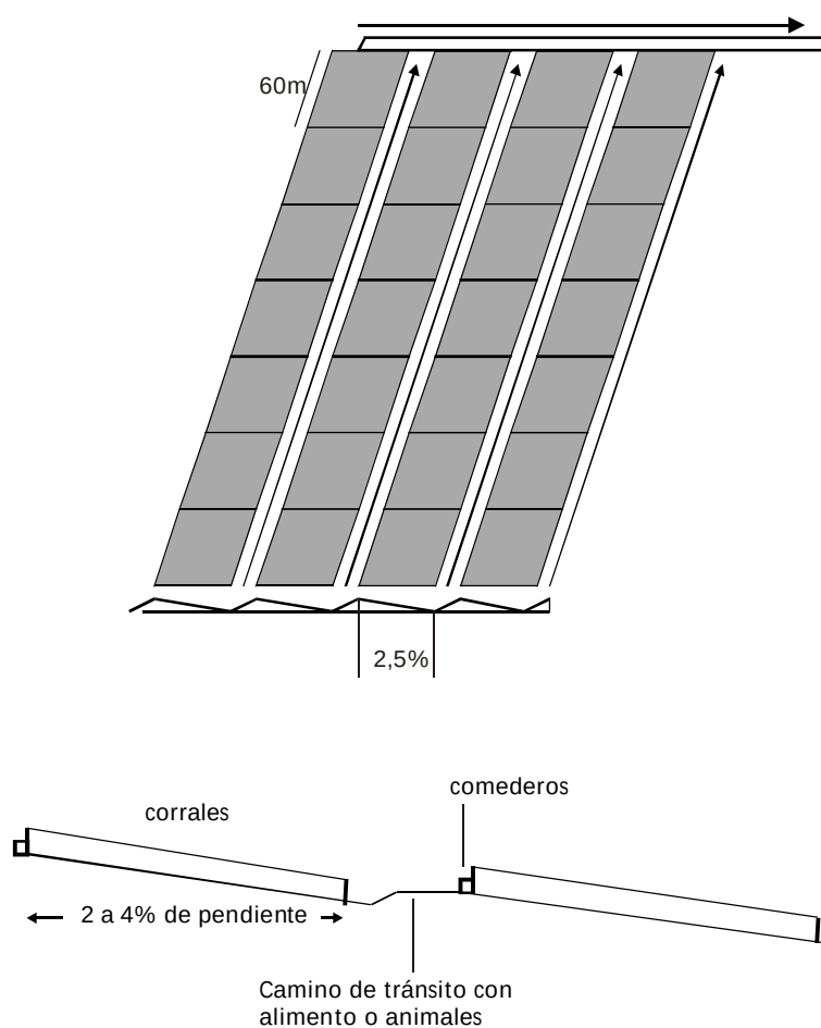
Diseño y ubicación espacial de los corrales
